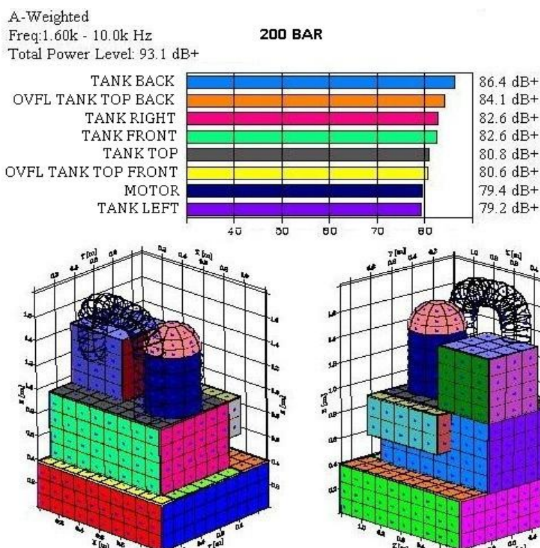
Rys. 5: Ranking poziomów mocy akustycznej dla poszczególnych powierzchni
