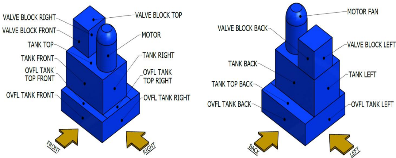
Rys. 4. Nazwy poszczególnych powierzchni modelu agregatu hydraulicznego
