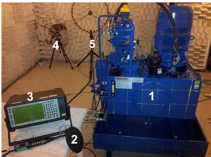
Rys. 2. 1- Agregat hydrauliczny, 2-Sonda dwumikrofonowa 3548 B&K, 3-Analizator 2144 B&K, 4- Kamera akustyczna Noise Inspector CAE, 5- Kamera akustyczna GFaI.
