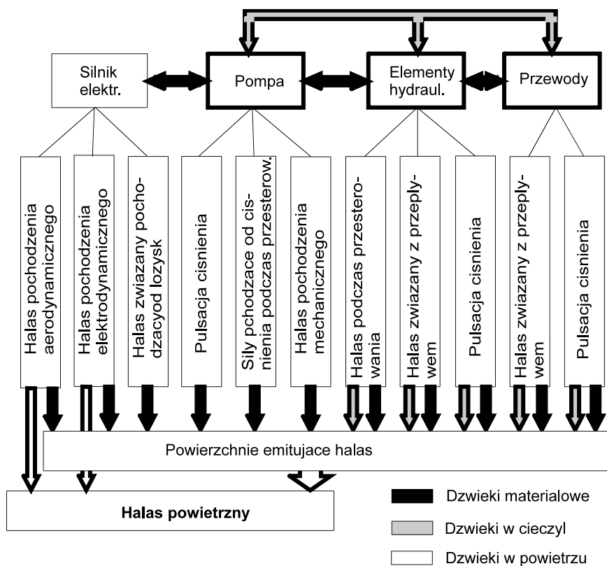
Rys. 1. Przyczyny powstawania hałasu w układach hydraulicznych
