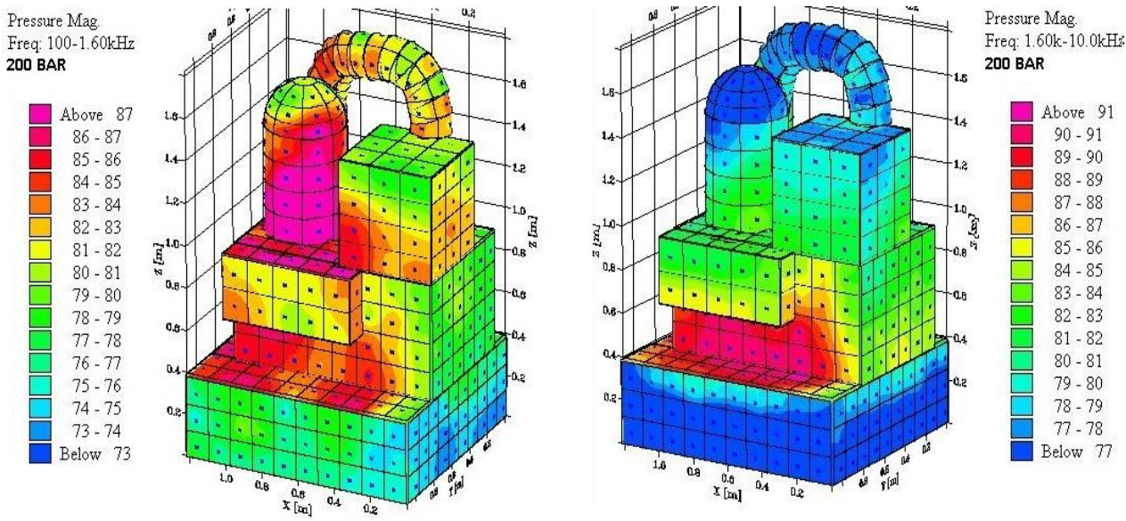
Rys. 3. Mapy ciśnienia akustycznego – widok tylnej części agregatu hydraulicznego
