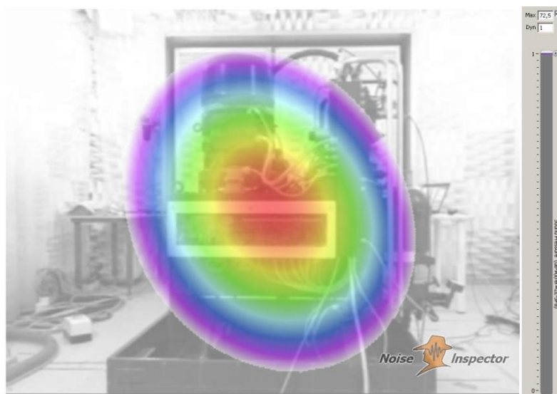
Rys. 6. Zdjęcie wykonane kamerą. Ciśnienie 200 bar – Zakres częstotliwości (0,1-1,6) kHz Fig. 6. Acoustic Photo. Operating pressure 200 bar. Frequency range (0,1-1,6) kHz
